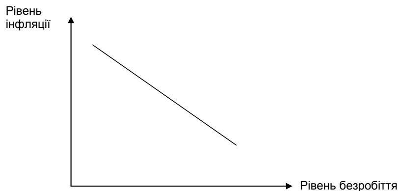
Рис. 2. Крива Філіппса
